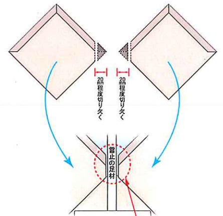
上ハぜが雪止の足材に重ならないようにする
