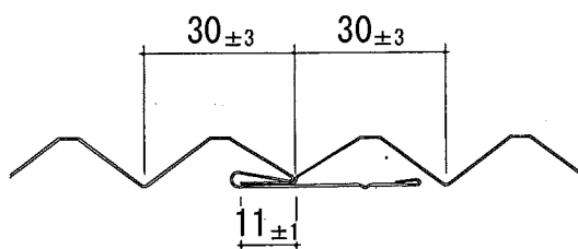
嵌合部
