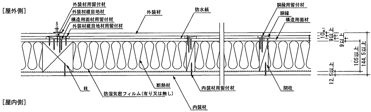
①外装材横張
