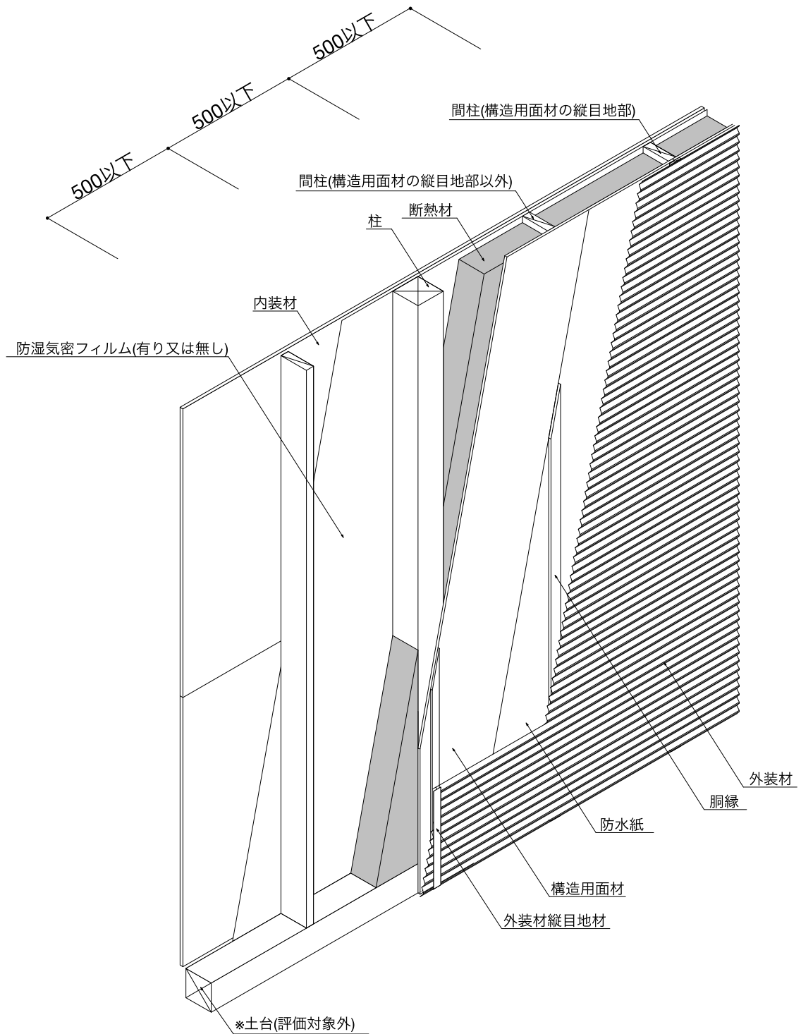
①外装材横張
