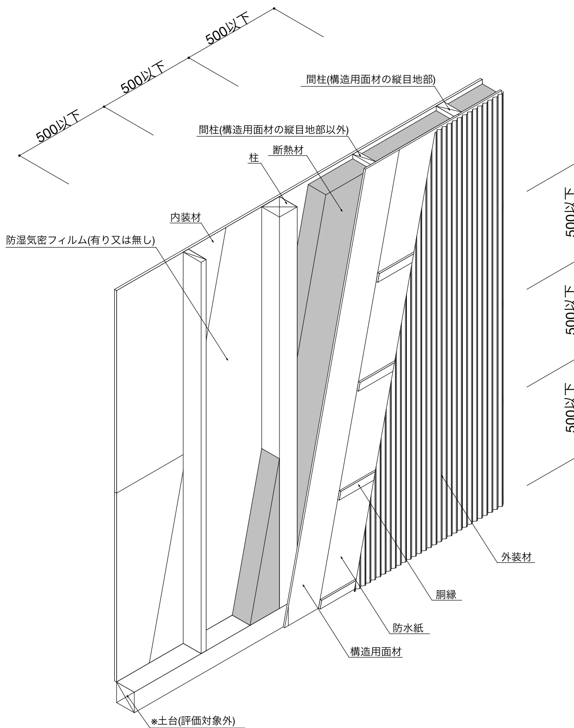
透視図
